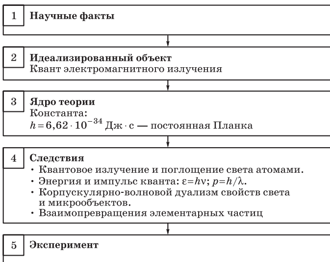
Рис. 14. СЛС «Элементы квантовой физики»
