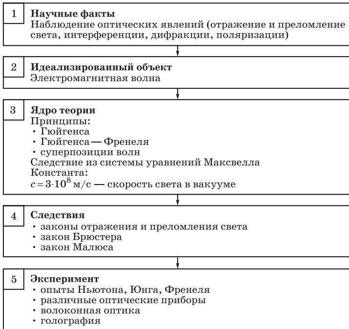
Рис. 11. Волновая оптика
