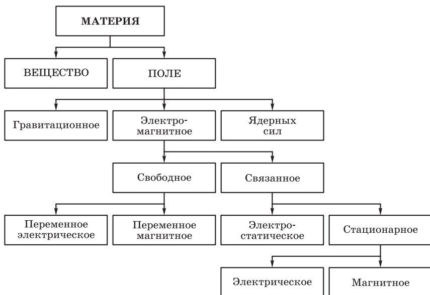
Рис. 10. Этапы изучения полей
