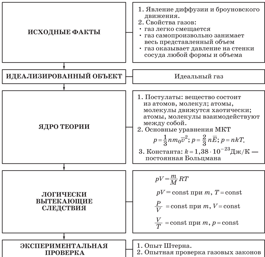
Рис. 5. Основы МКТ
