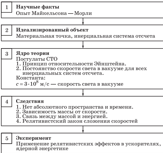
Рис. 12. Специальная теория относительности (СТО)
