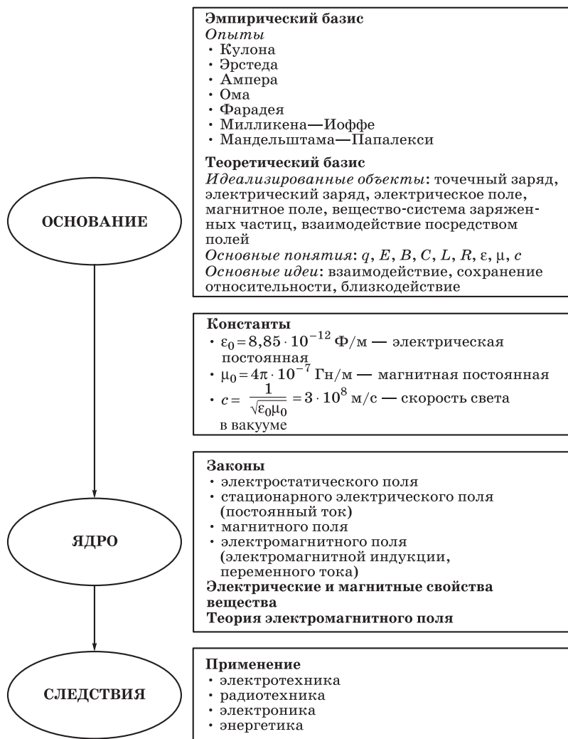
Рис. 8. Структура и содержание электродинамики
