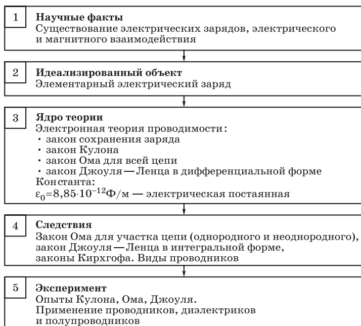
Рис. 9. Основы электродинамики
